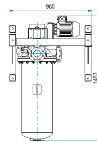
Dimensions OptiFil-M-250-0720
